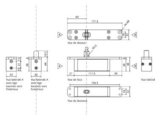
Pivot supérieur
