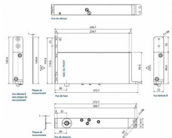
Pivot inférieur
