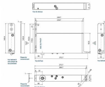
Pivot inférieur
